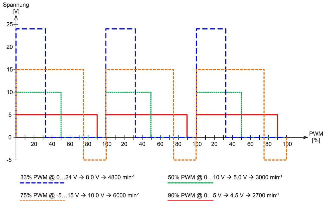
Abbildung 3-8 Eingang «Drehzahlsollwert» – Beispiele möglicher PWM-Ansteuerungen
