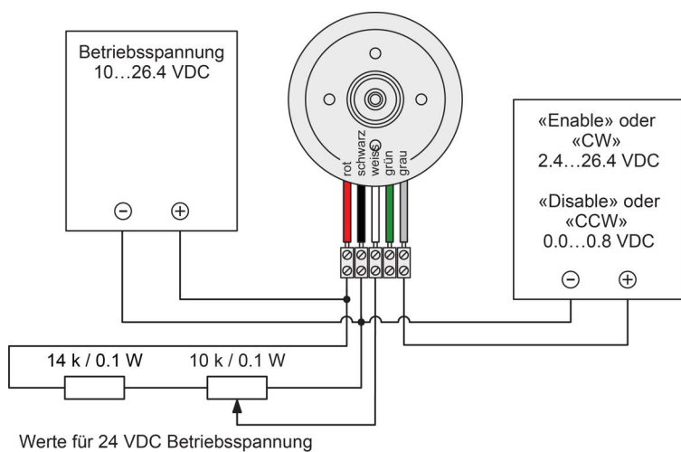
Abbildung 4-14 Drehzahlsollwert über externes Potentiometer und «Enable» oder «Drehrichtung» mit externer Spannungsquelle
