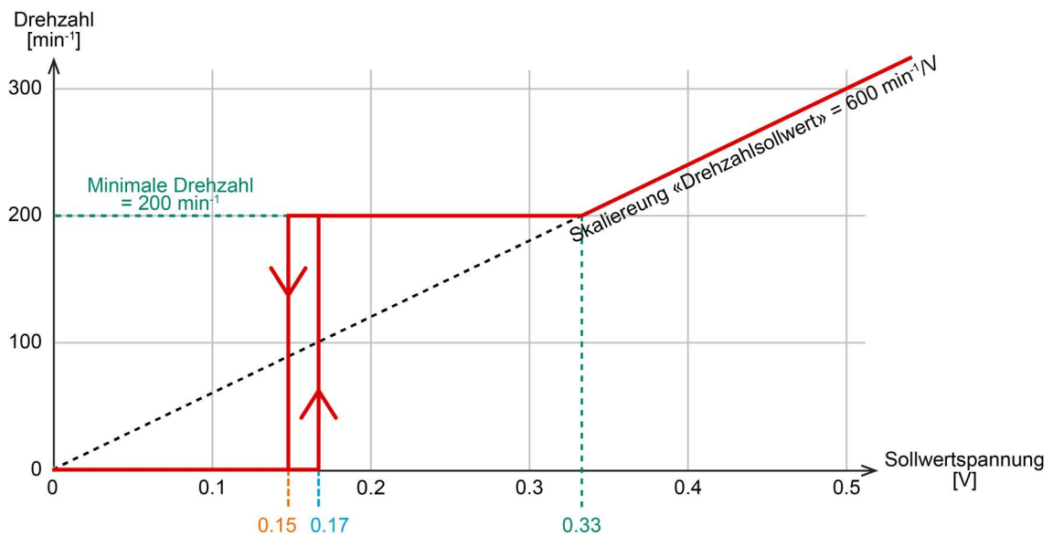
Abbildung 3-7 Eingang «Drehzahlsollwert» – Ein- und Ausschalthysterese (Detail)
