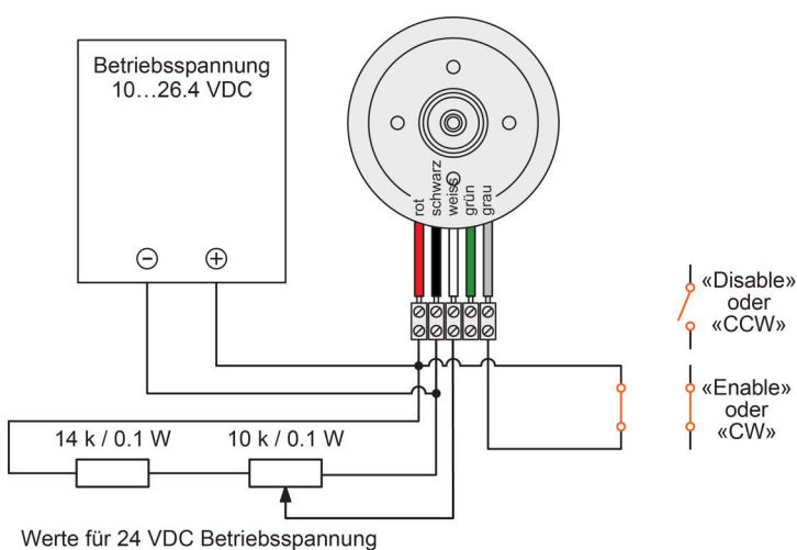
Abbildung 4-15 Drehzahlsollwert über externes Potentiometer und «Enable» oder «Drehrichtung» mit potentialfreiem Kontakt
