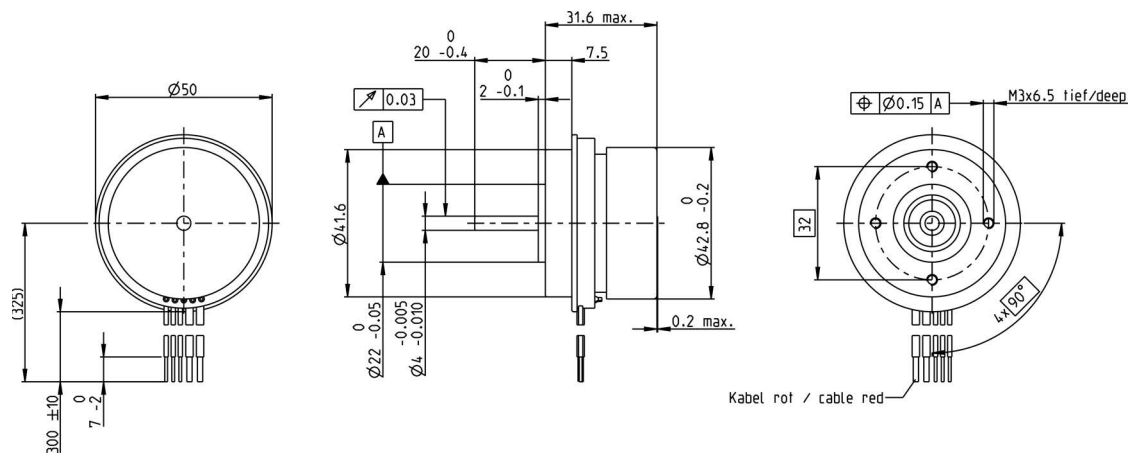
Abbildung 2-1 30 Watt-Ausführung / IP00 – Massbild [mm]
