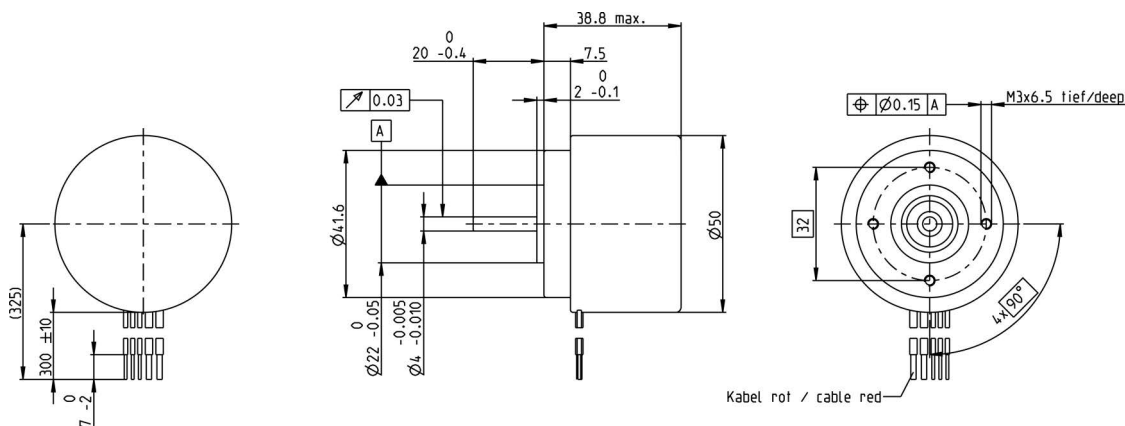
Abbildung 2-4 50 Watt-Ausführung / IP40 – Massbild [mm]
