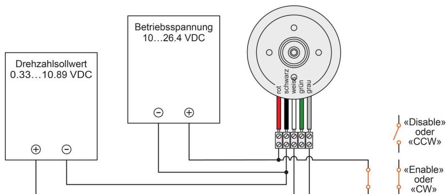
Abbildung 4-13 Drehzahlsollwert über externe Spannungsquelle und «Enable» oder «Drehrichtung» mit potentialfreiem Kontakt
