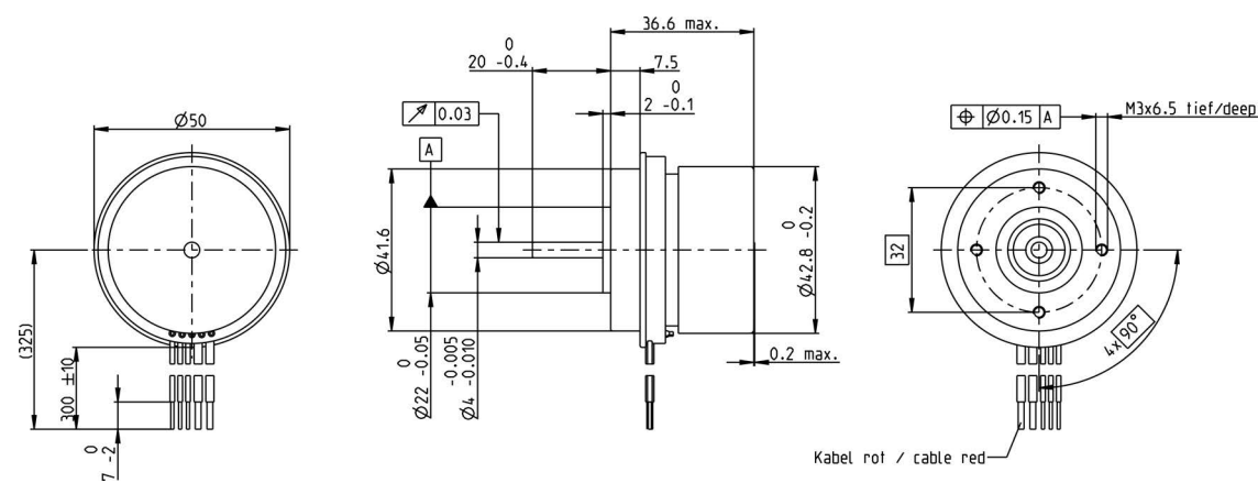
Abbildung 2-3 50 Watt-Ausführung / IP00 – Massbild [mm]
