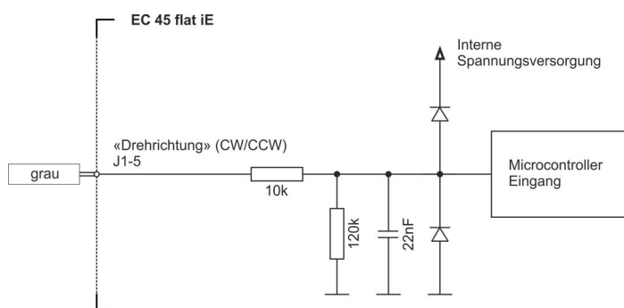
Abbildung 3-10 Eingang «Drehrichtung» – interne Beschaltung
