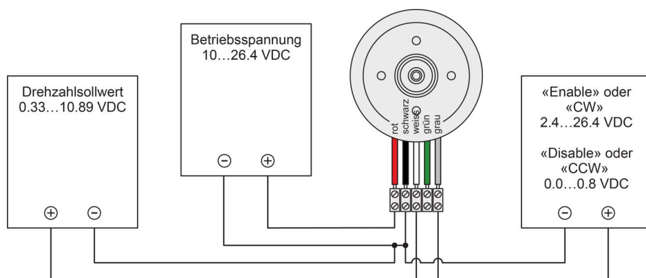
Abbildung 4-12 Drehzahlsollwert und «Enable» oder «Drehrichtung» über externe Spannungsquelle
