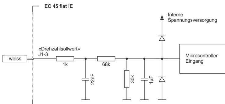
Abbildung 3-5 Eingang «Drehzahlsollwert» – interne Beschaltung
