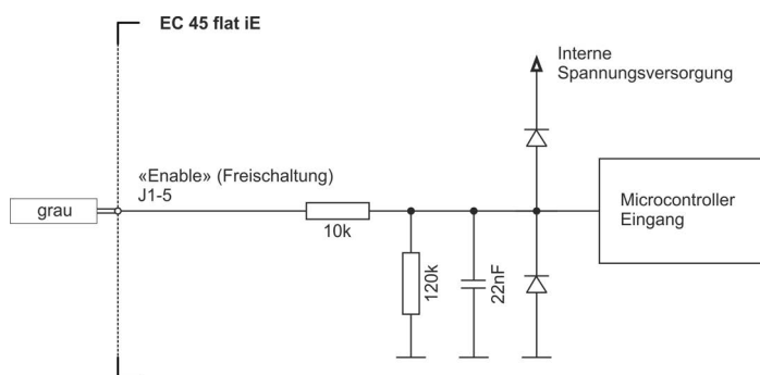
Abbildung 3-9 Eingang «Enable» – interne Beschaltung
