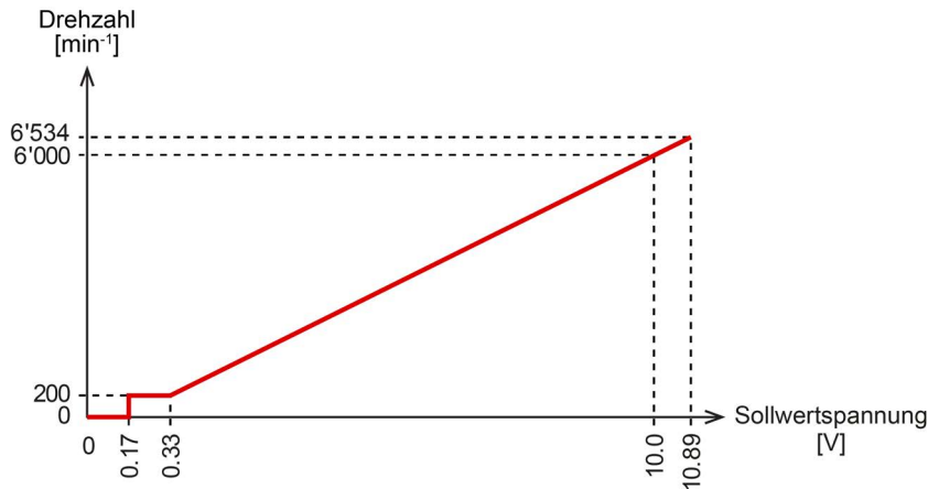
Abbildung 3-6 Eingang «Drehzahlsollwert» – Kennlinie
