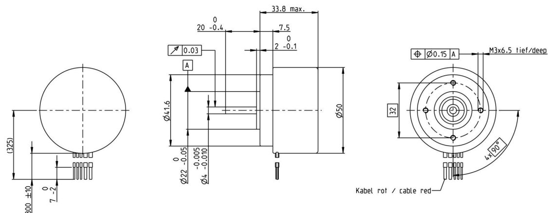
Abbildung 2-2 30 Watt-Ausführung / IP40 – Massbild [mm]
