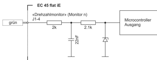
Abbildung 3-11 Ausgang «Drehzahlmonitor» – interne Beschaltung
